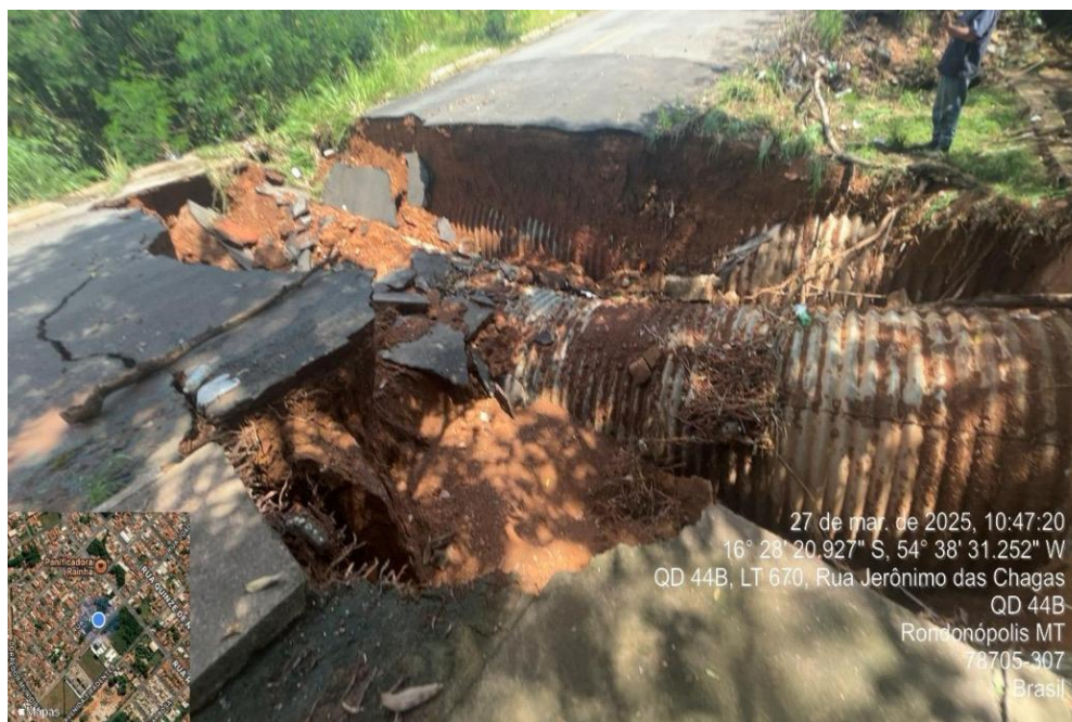
Imagem 1 - Vista geral do trecho da via que sofreu colapso, expondo a tubulação de drenagem e o solo erodido. Detalhes da erosão formada e da instabilidade do pavimento
