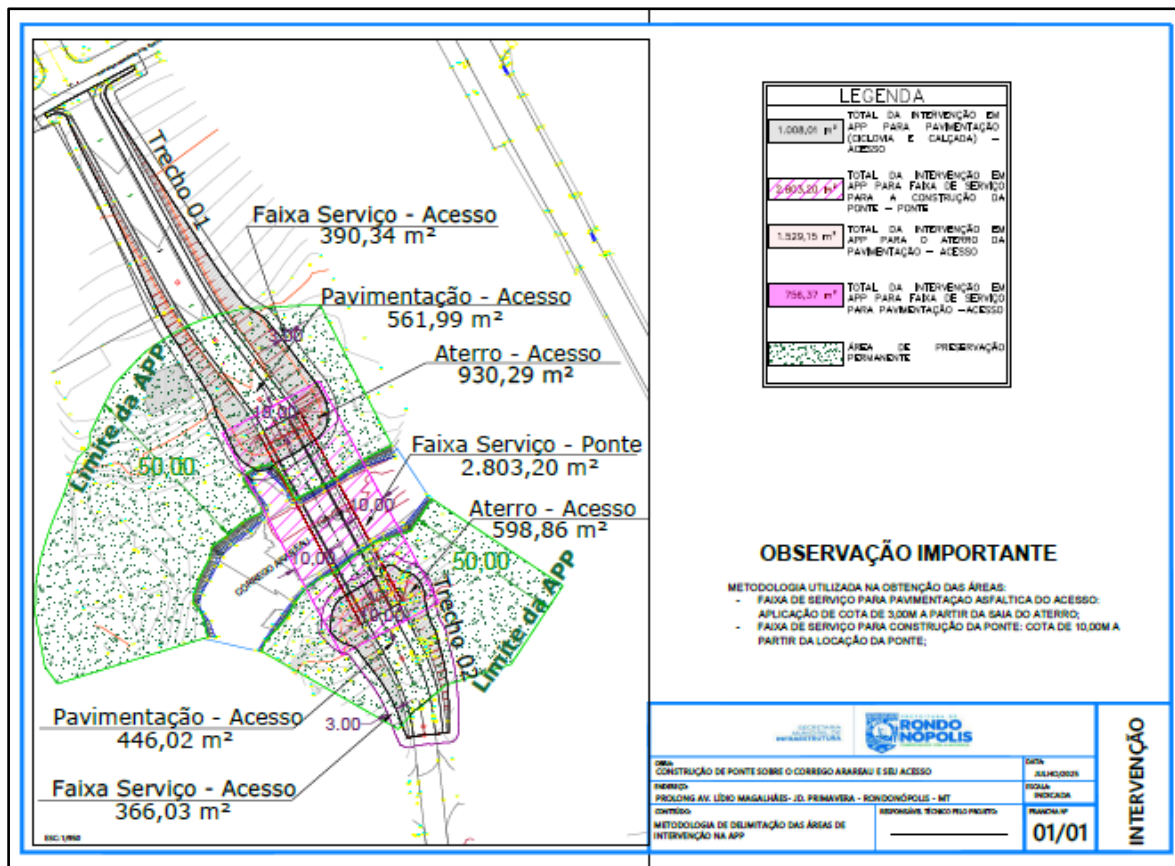
Figura 02 - planta de intervenção
