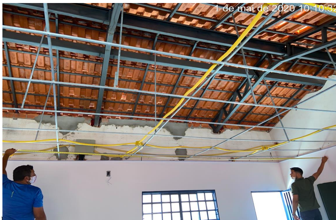
Imagem 03 – Estrutura de fixação do forro sem a devida acarração no madeiramento, o que ocasionou envergamentos.
