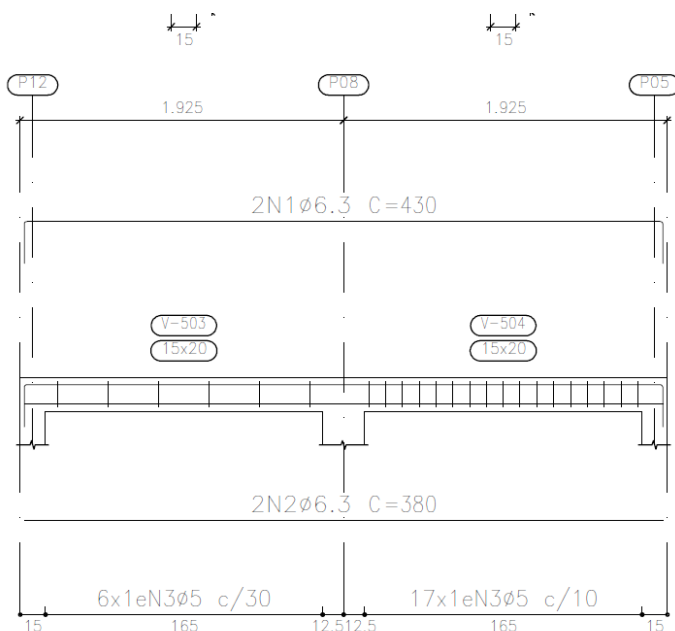
NÍVEL DA VIGA DE RESPALDO, VISUALIZANDO OS PILARES EM CORTE
