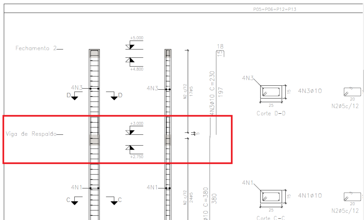
NÍVEL DA VIGA DE RESPALDO, VISUALIZANDO OS PILARES EM CORTE
